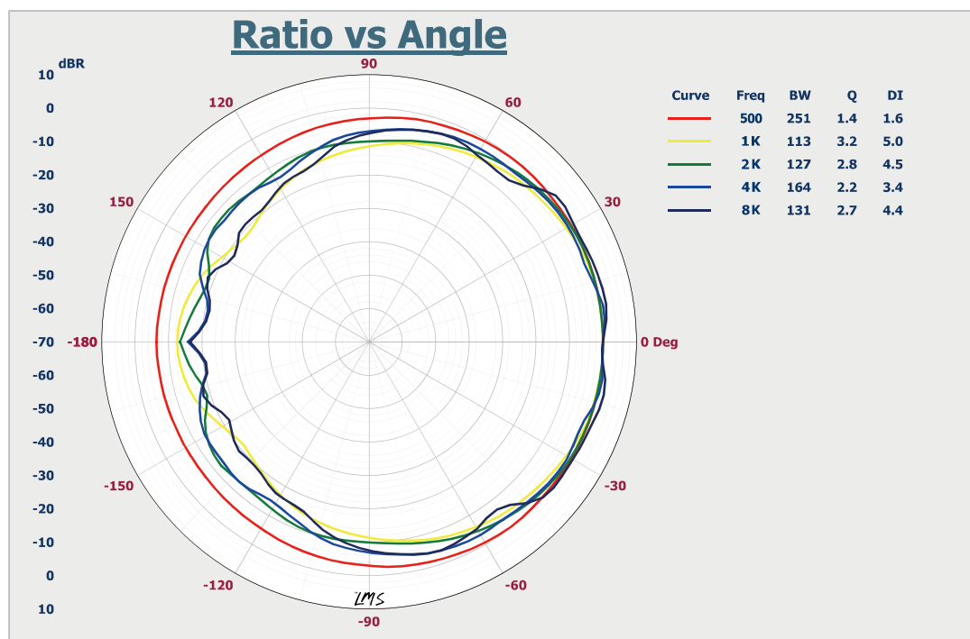
Круговая диграмма направленности громкоговорителя LPA-3C
